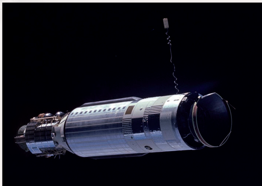
Орбитальный блок Agena, использовавшийся для отработки операций по стыковке в ходе миссии Gemini 8 в марте 1966 г.
